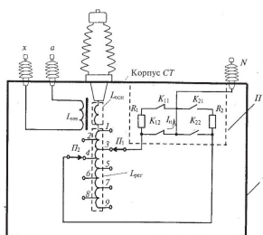
Рис. 1. Основные цепи фазы трансформатора.
