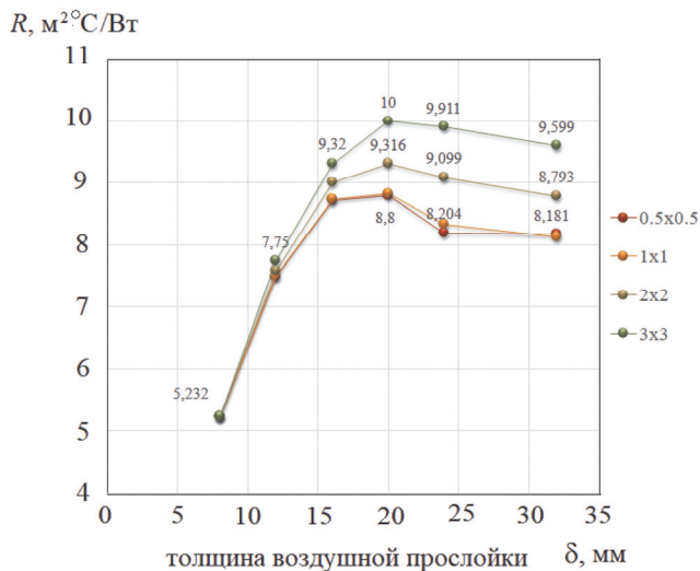
Рис. 1. Термические сопротивления ограждающей конструкции
