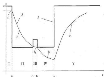
Рис. 2. Диаграммы фазного тока РПН.
