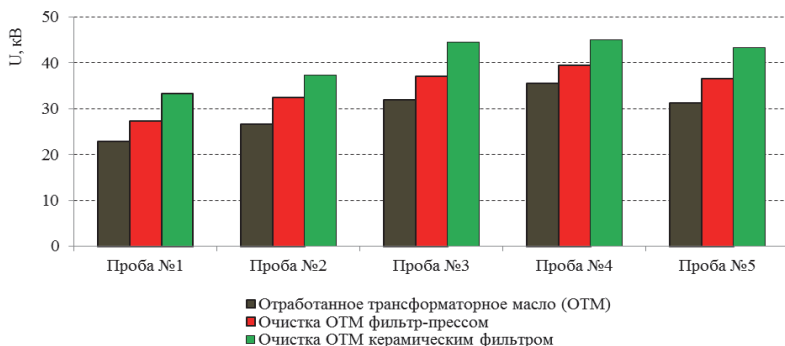
Рис. 1. Средние арифметические значения пробивных напряжений отработанных трансформаторных масел до и после очистки
