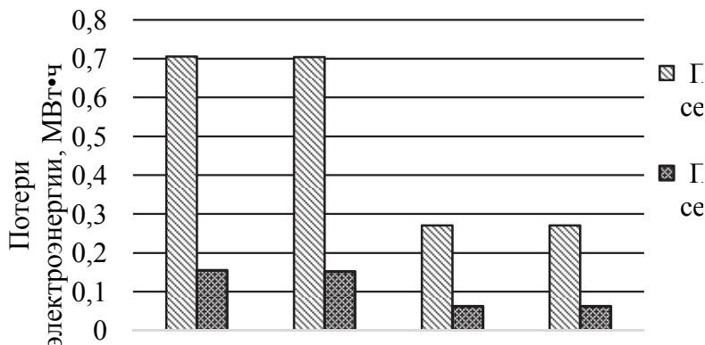
Рис. 1. Результаты расчетов в сетях 10 и 20 кВ
